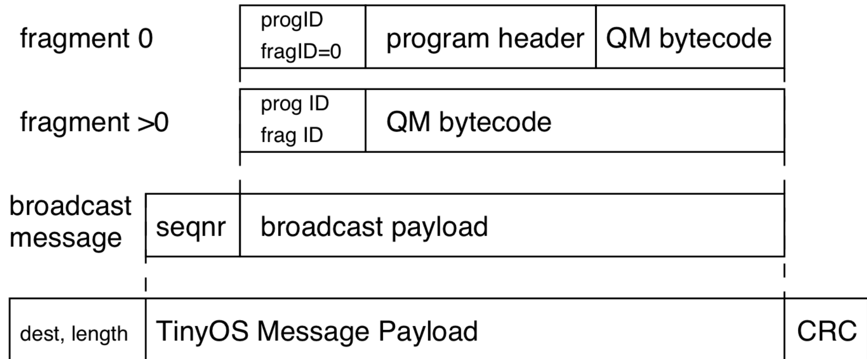
TinyOS Message
